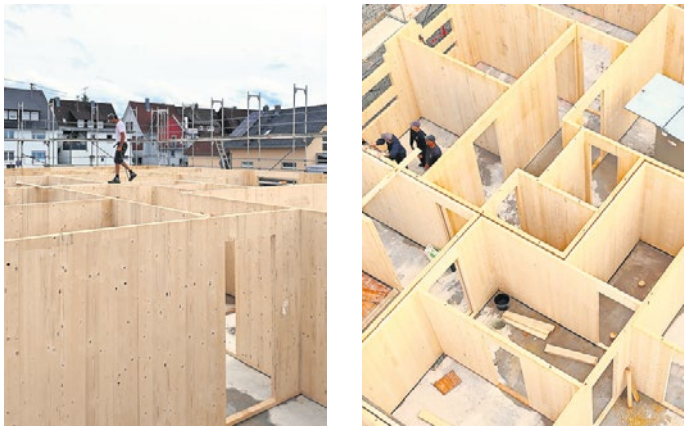
Schönes Projekt: ein Mehrfamilienhaus mit acht Wohneinheiten aus Brettsperrholz. Foto: Hess
